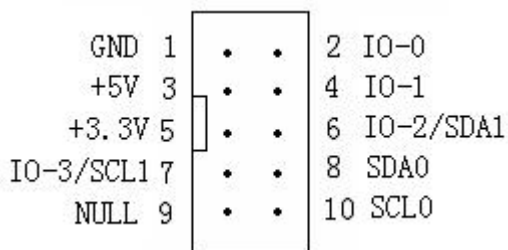
图 2 适配器对外接口（针式）
