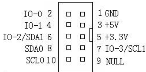
图 3 适配器对外排线接口
