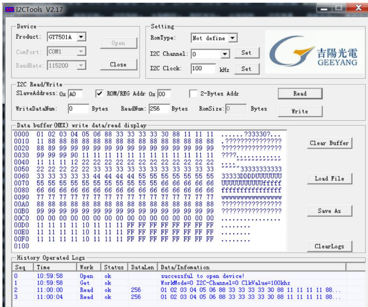
图 3 I2CTools 主界面
